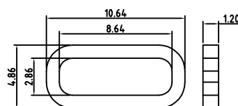
壳及接触尺寸
