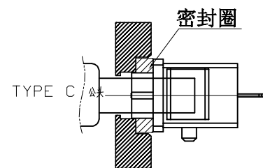
组装示意图
