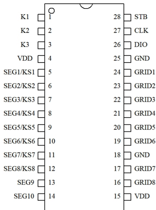
1638 28SOP/SSOP
