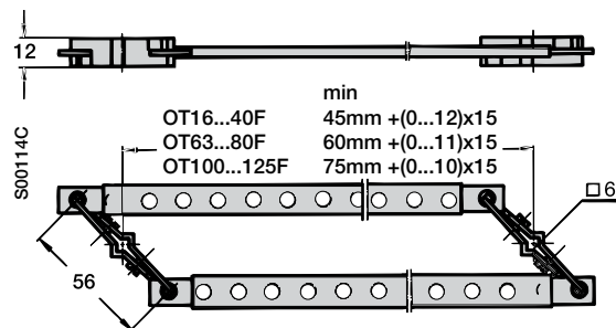
OTZW 8
