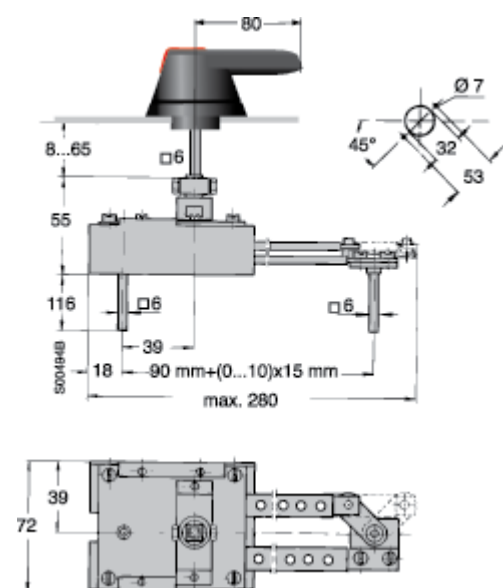
OESAZW1
