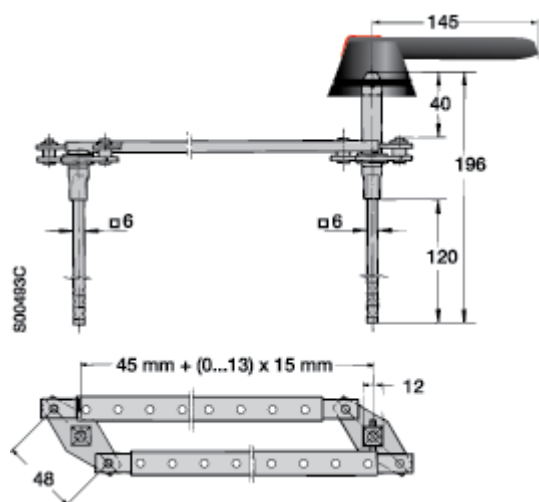
OESAZW 2
