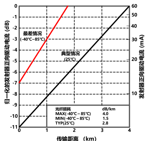
图 8 配合 62.5/125μm 芯径光纤 NRS1414xx/HFBR-2412 传输距离极限
