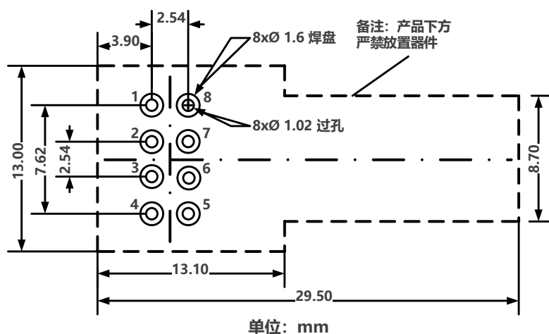
图 5 PCB Layout 设计推荐尺寸图 (俯视图)
