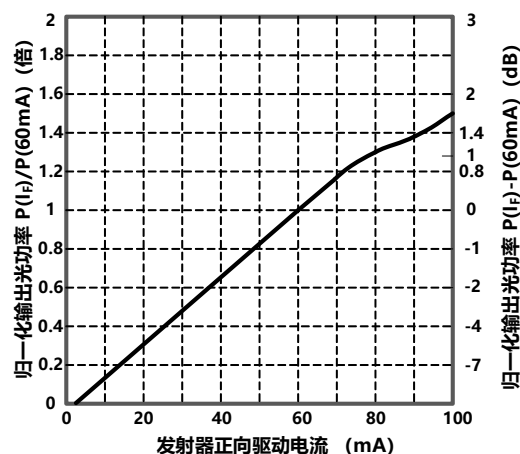
图 4 正向导通电流与归一化输出光功率曲线
