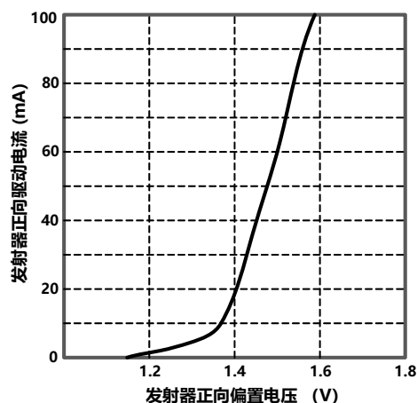
图 3 正向偏置电压与正向驱动电流曲线
