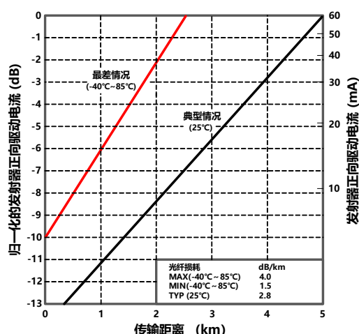
图 7 配合 62.5/125μm 芯径光纤 NRS1414xx/2412xx 传输距离极限
