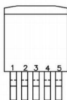
TO263-5L
