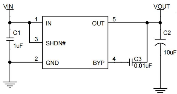
图 2 LKP2872ST-18/30/33/5 典型应用电路图
