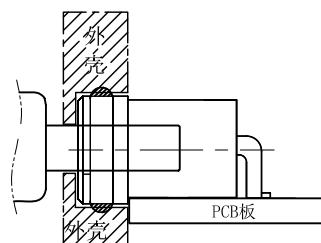
组装示意图
