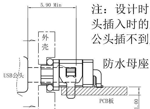
组装示意图
