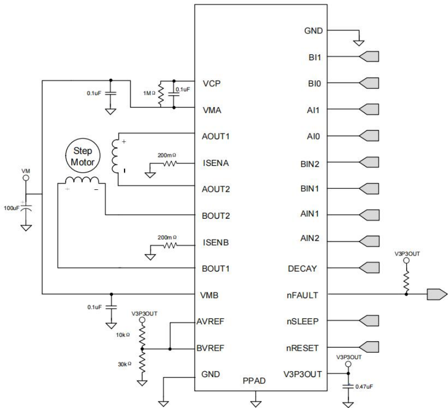
图 6 典型应用电路
