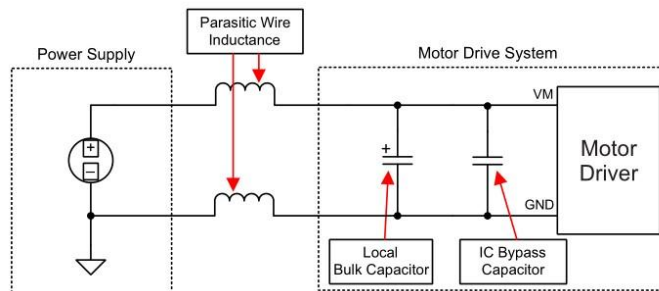
图 8 外置电源电机驱动系统的设置
