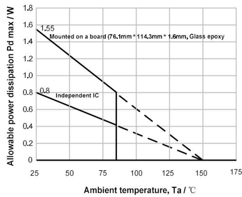
图 2 ETSSOP28 with PAD 额定参数曲线图
