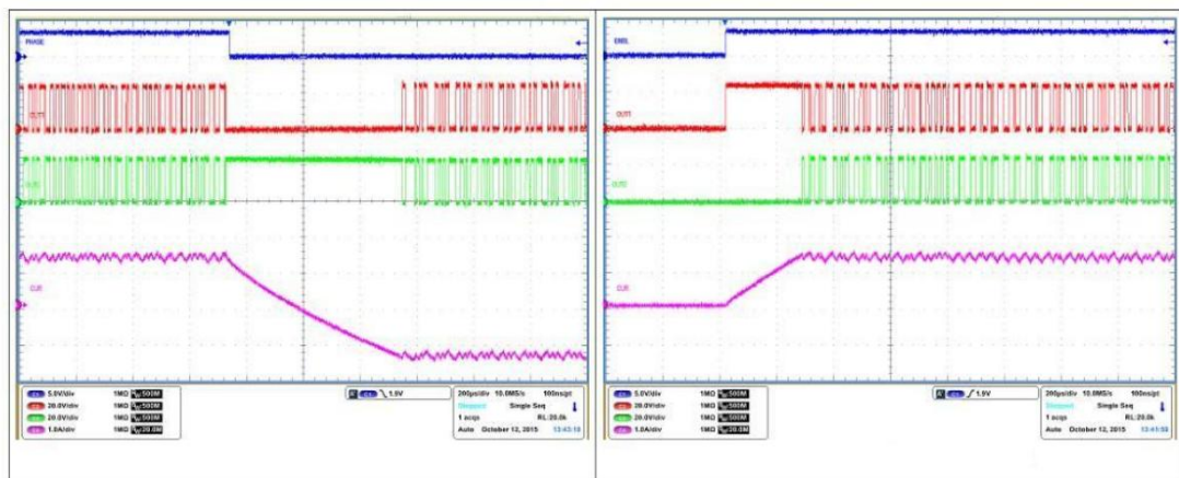
图 7 应用波形图
