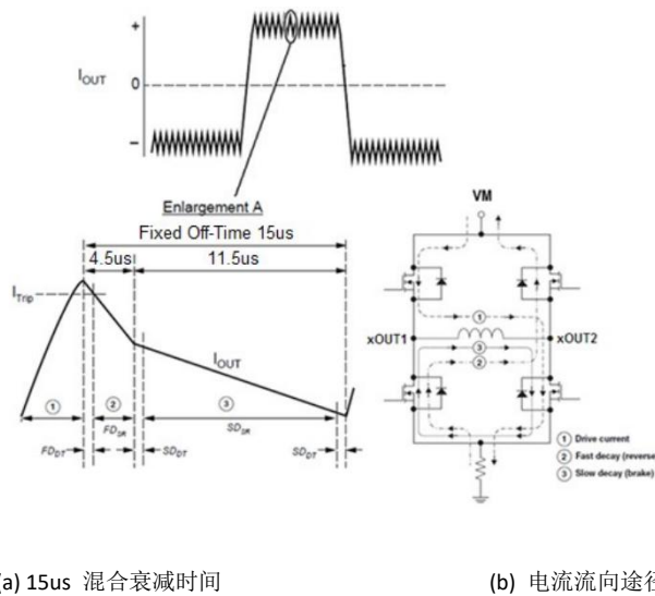
图 5 混合衰减模式
