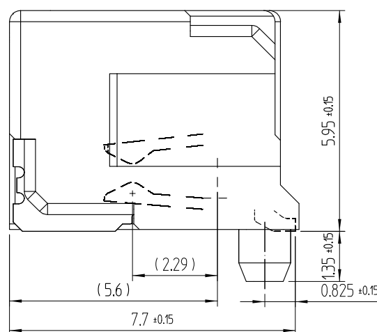
A-A (7:1)
