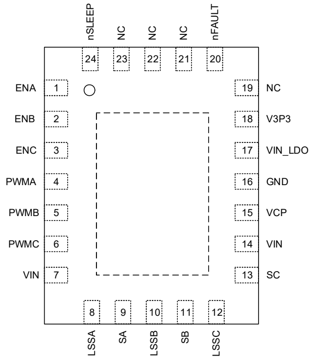
图 2 脚位图
