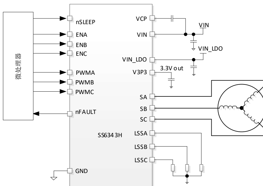
图 1 典型应用原理图
