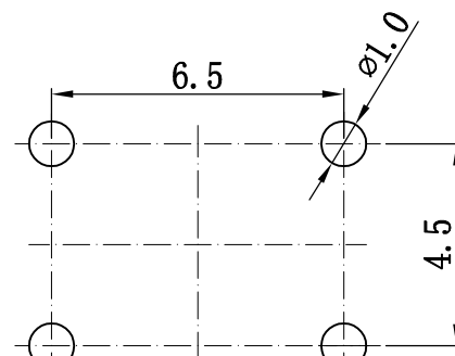
PCB板开孔尺寸( \pm 0.1 )
