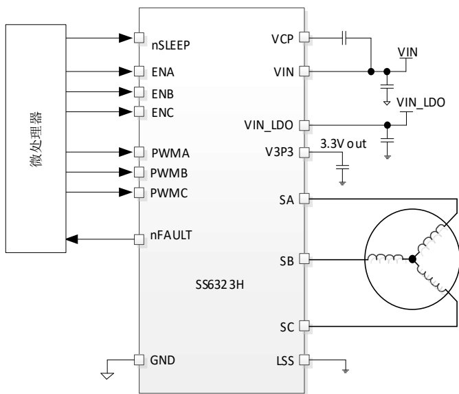
图 1 典型应用原理图
