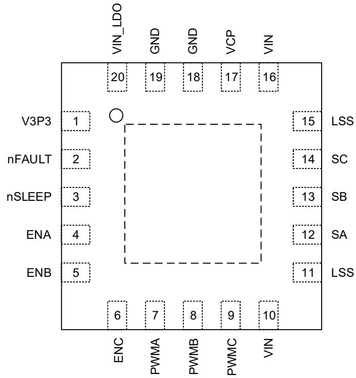
图 2 脚位图
