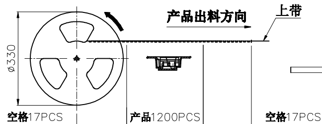
① 产品入载带示意图
