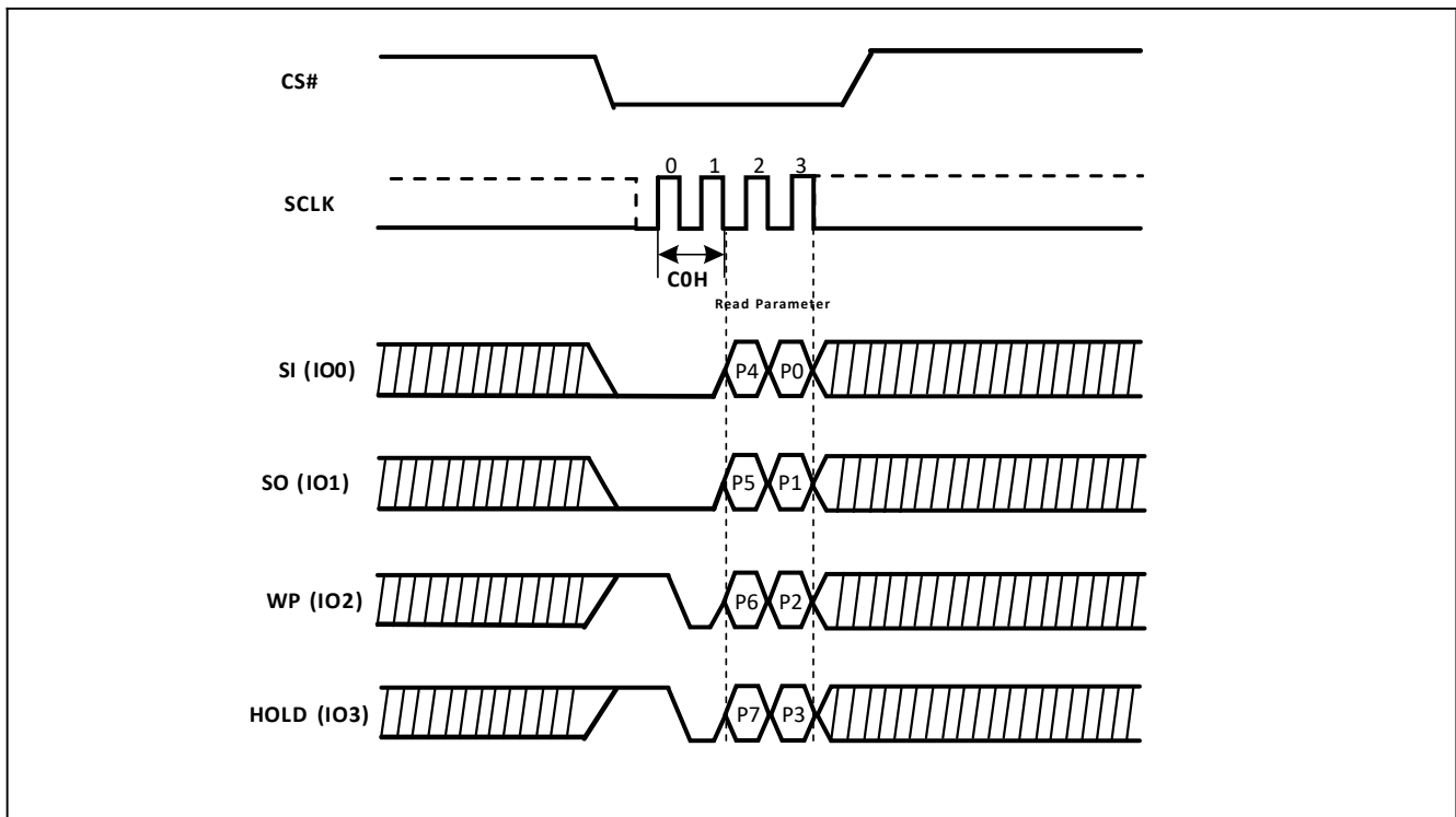
Figure-34. Set Read Parameters (QPI)
