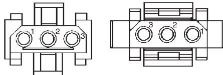
Receptacle
