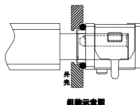
组装示意图
