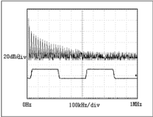
图11：传输20kHz信号时 TD3485-3.3-TD驱动器输出波形和FFT图
