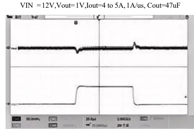
图5 1.0V 输出瞬态响应
