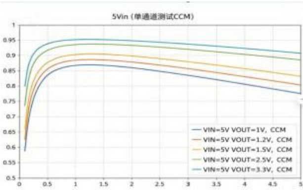
图 3 效率 VS 5VIN 负载电流
