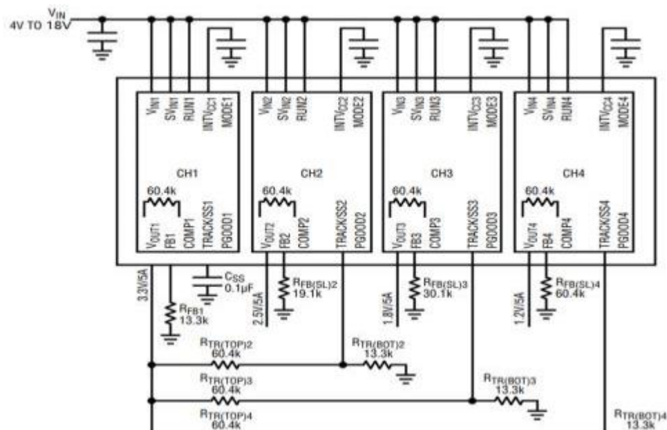
图 18 输出比例跟踪原理图
