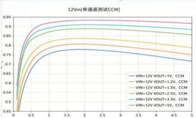
图4效率 VS 12VIN 负载电流
