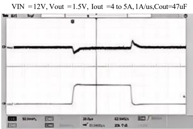
图6 1.0V 输出瞬态响应
