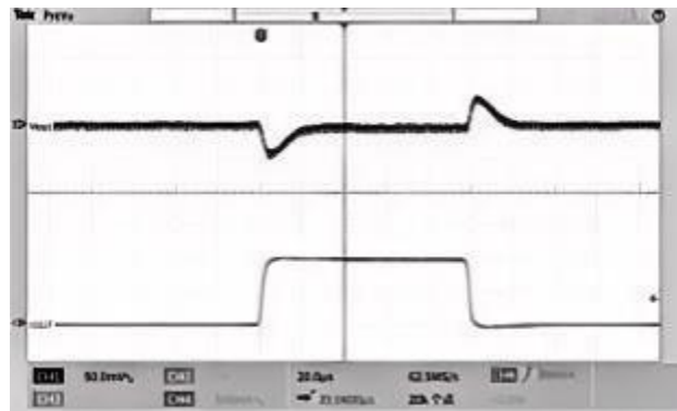
图8 3.3V输出瞬态响应
