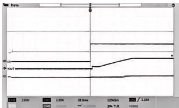
图14 空载启动
