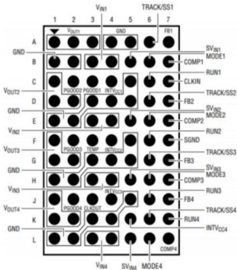
图2 引脚示意图
