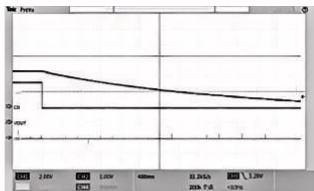
图15 空载关闭
