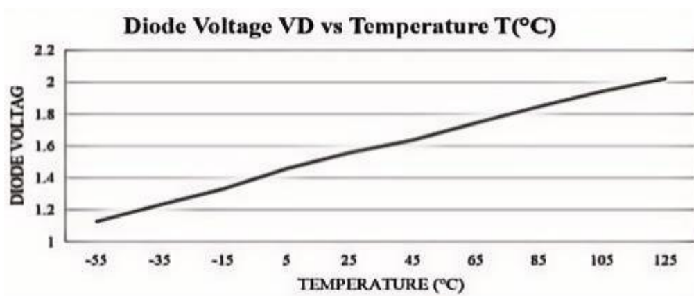
图16 温度检测: TEMP电压VS温度
