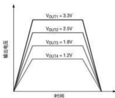
图 17 输出比例跟踪波形
