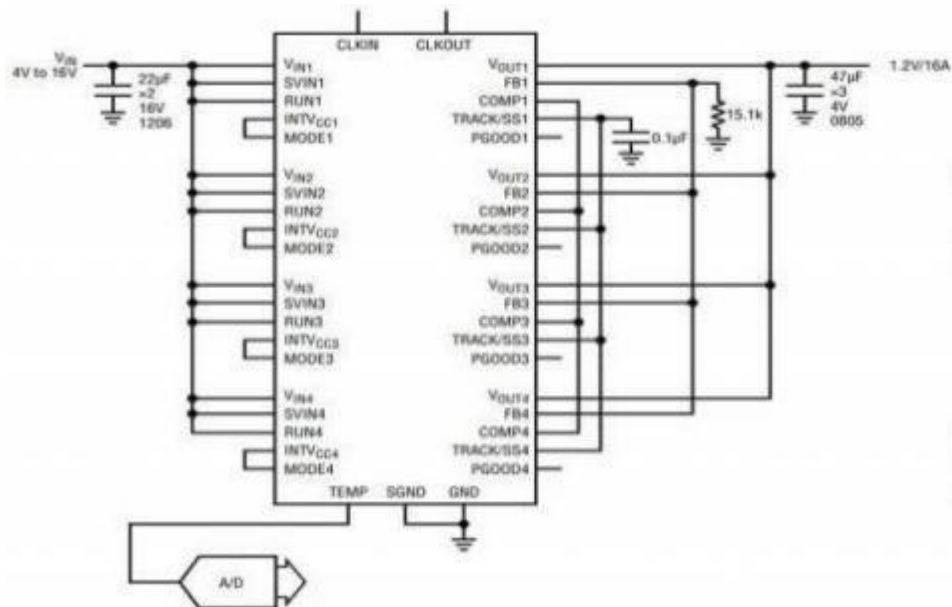
2 有温度监控功能的 4V~16V 输入、4 相、1.2V、16A 设计
