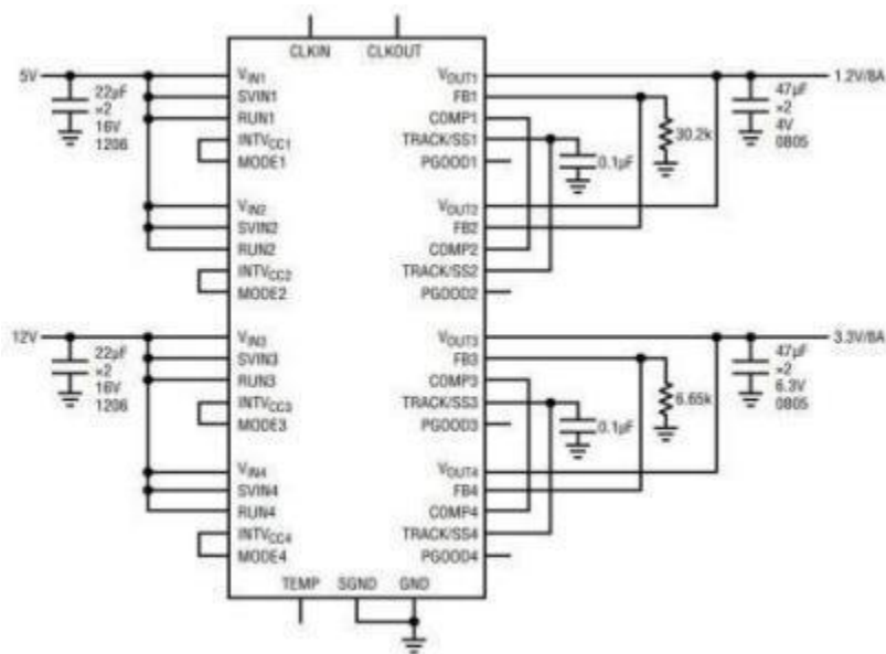
图 21 12V 和 5V 两个独立的输入轨，8A 输出 1.2V/8A 输出 3.3V
