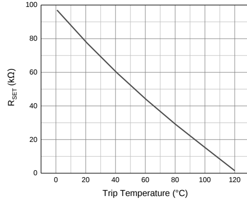
Rset 与触发温度的关系
