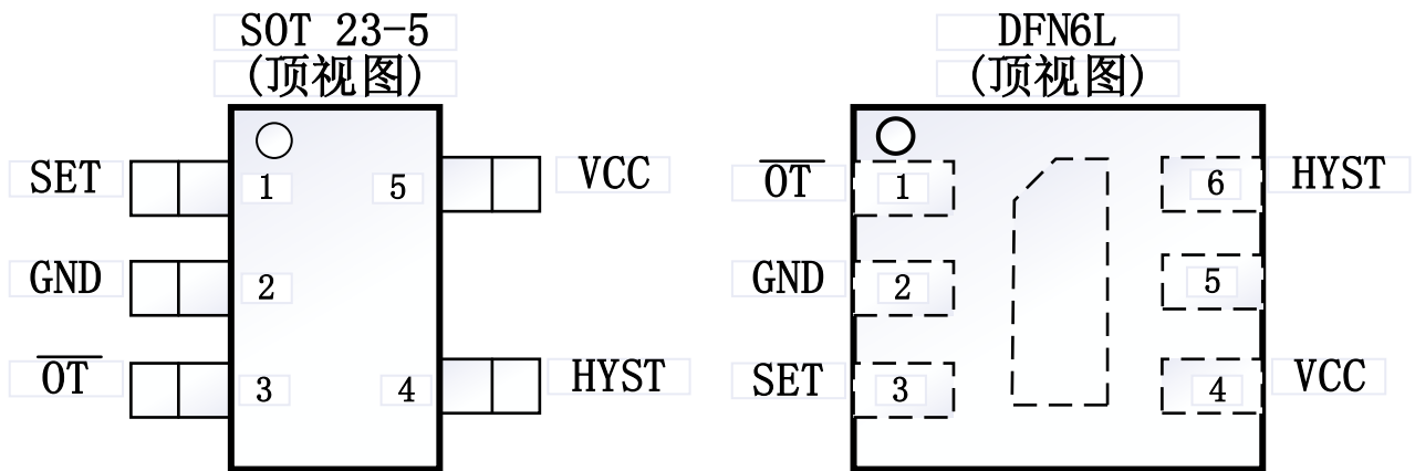
引 脚 功 能
