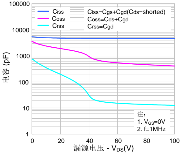
图7. 电容特性
