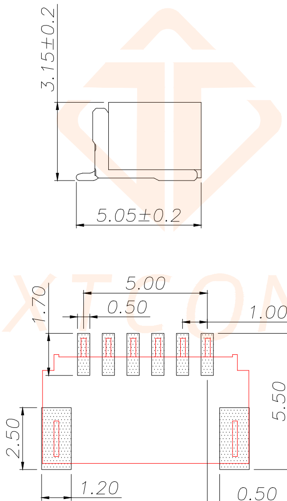
P.C.B LAYOUT
