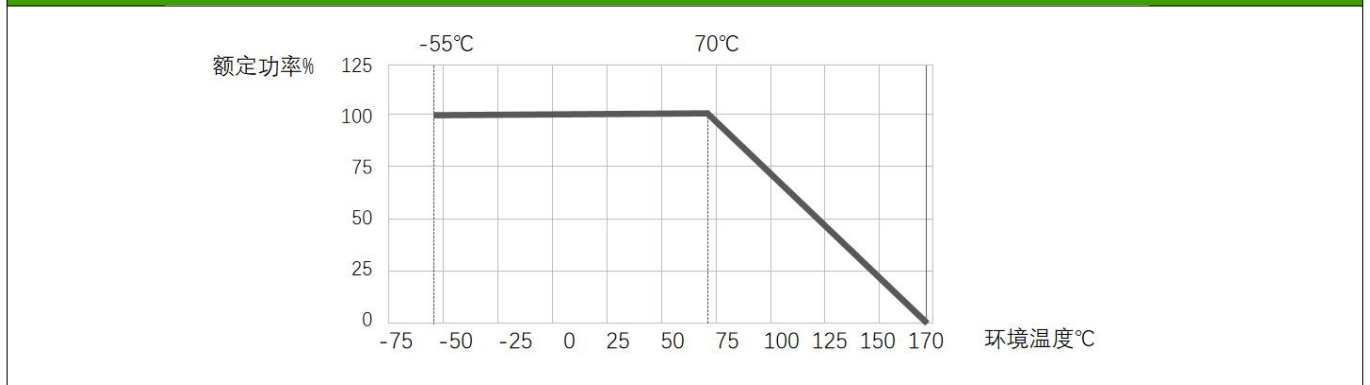
操作温度范围-55~+170℃电阻温度达到70℃时降功率示意图
