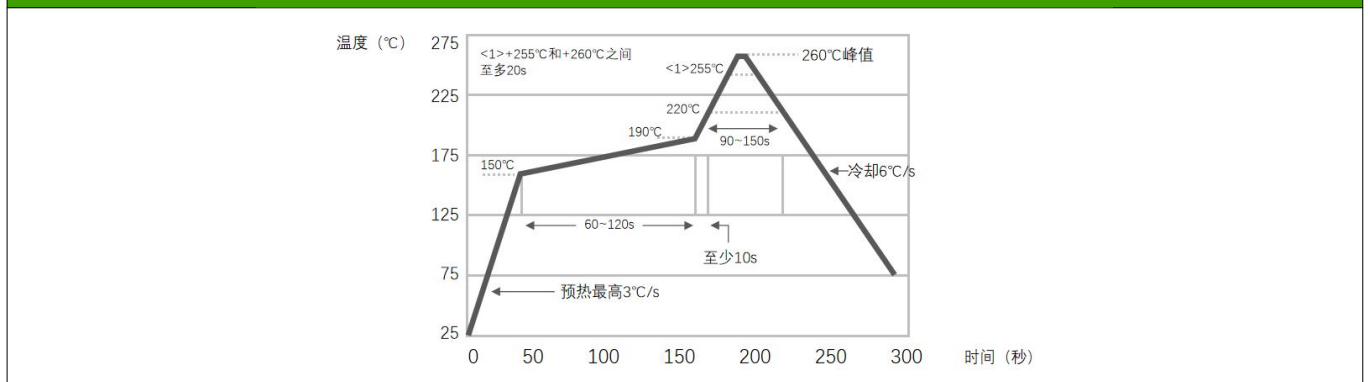
回流焊温度曲线
