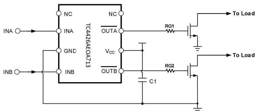
TC4426AEOA713反相典型应用电路图
