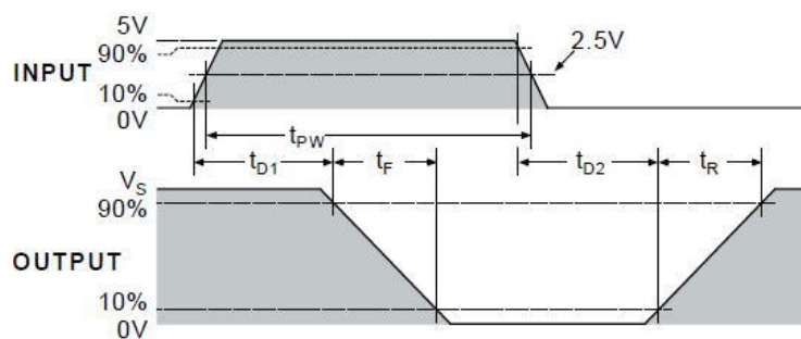
输入输出(反相)波形图
