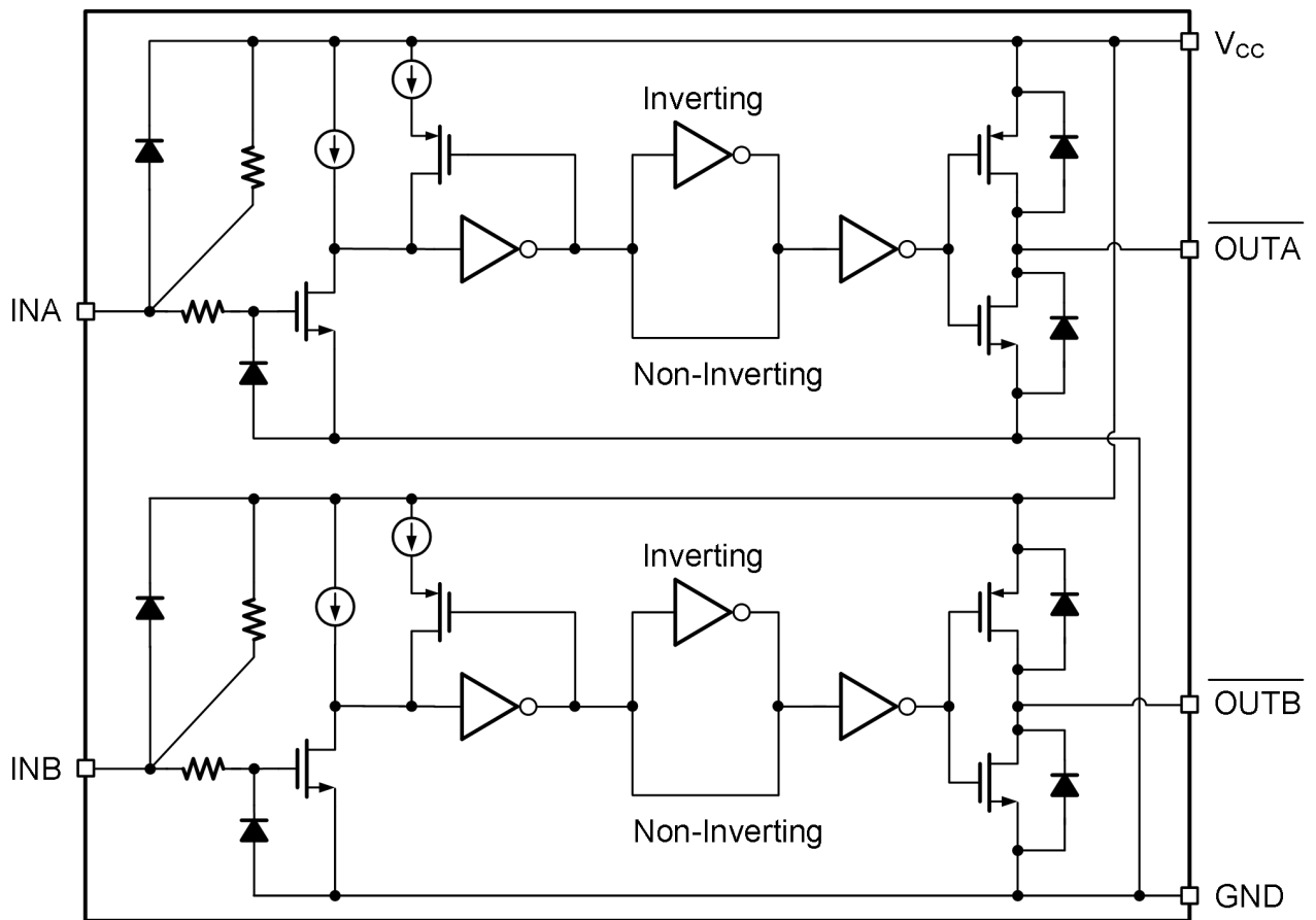
TC4426AEOA713功能框图
