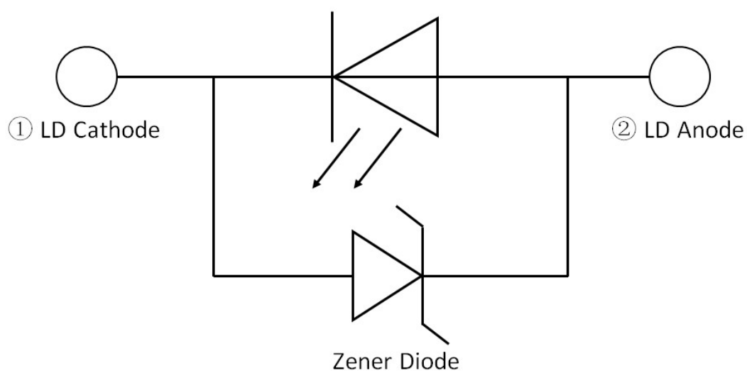
图 6-1 内部电路图
