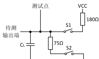
图 1 开关特性测试电路
