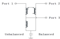
原理框图
