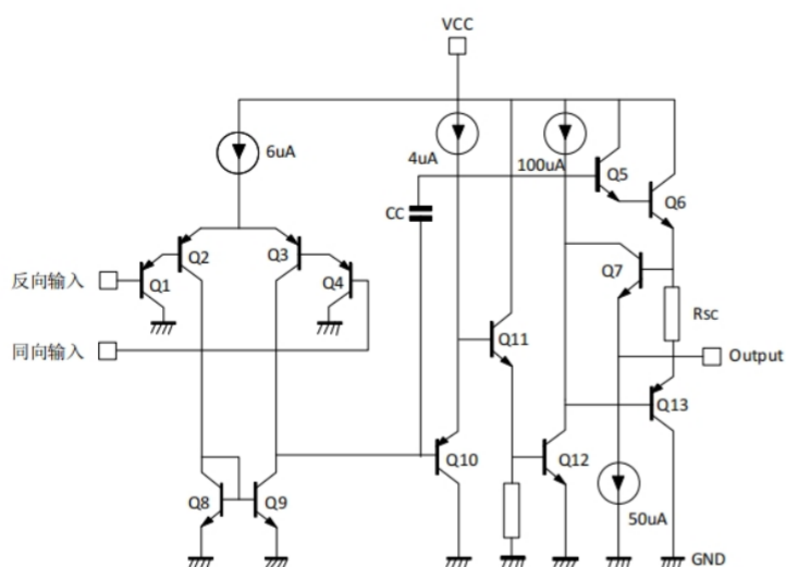
LM2904的内部原理图
