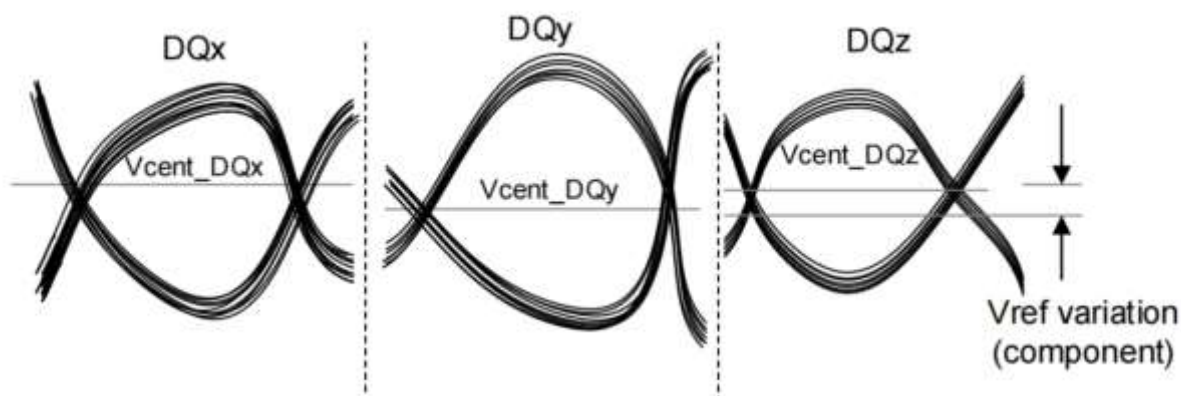
Figure 8-9 Across Pin Vref DQ Voltage Variation
