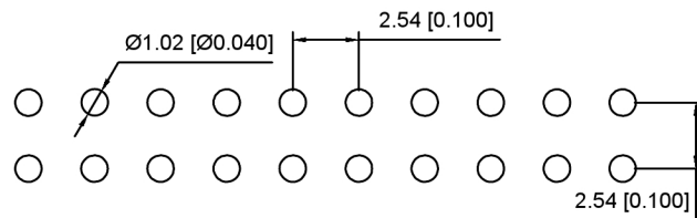
P.C.B LAYOUT
