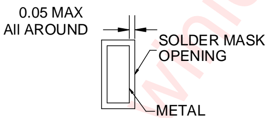
NON SOLDER MASK DEFINED
