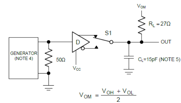
图 1 发送 V_{OH} 和 V_{OL}
