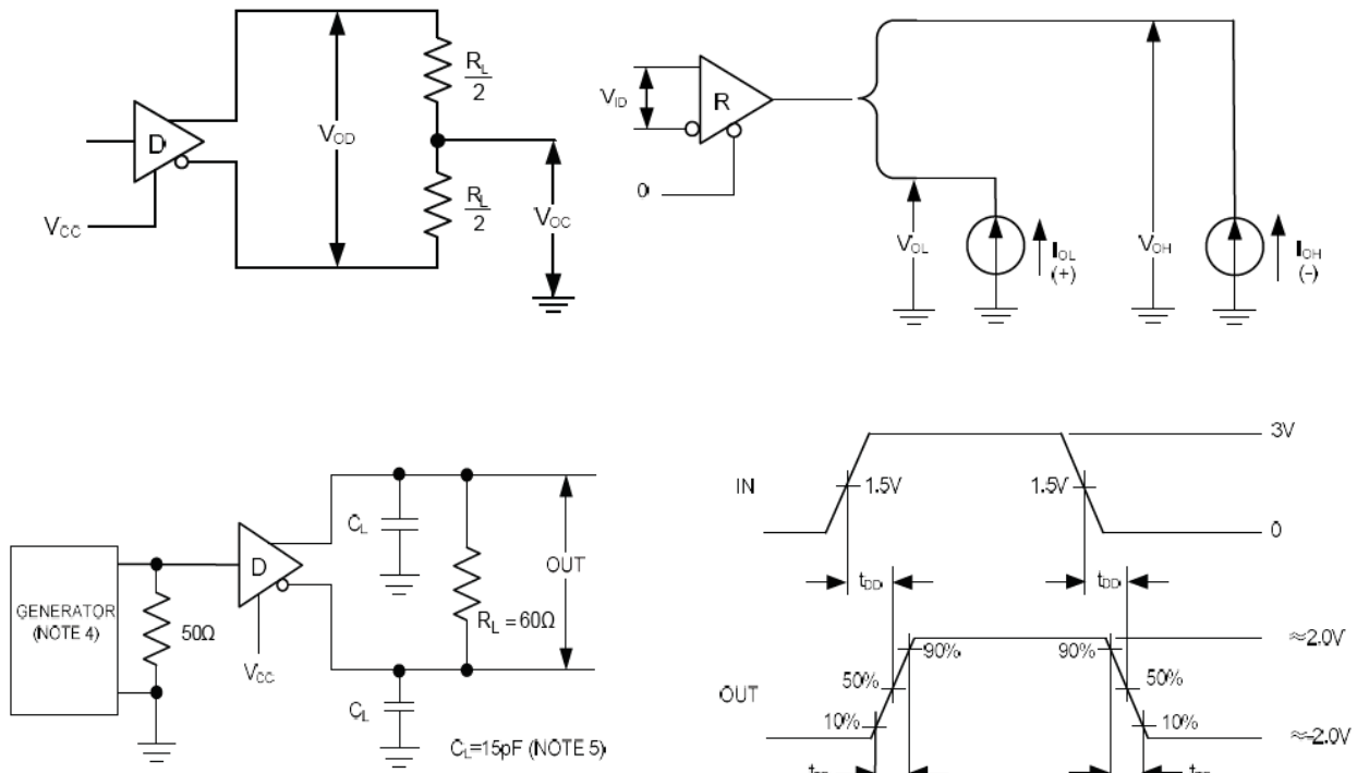
图 3 差分输出延时和转换时间
