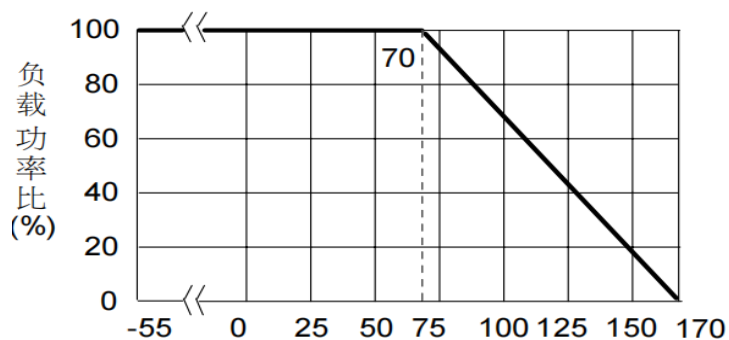
操作温度范围-55℃~+170℃电阻温度达到70℃时降功率示意图
