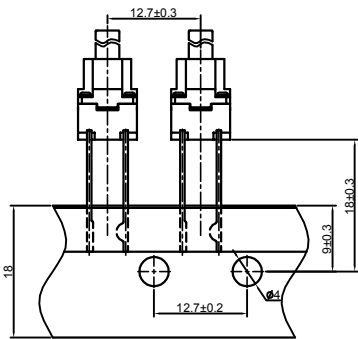
图1 编带图
