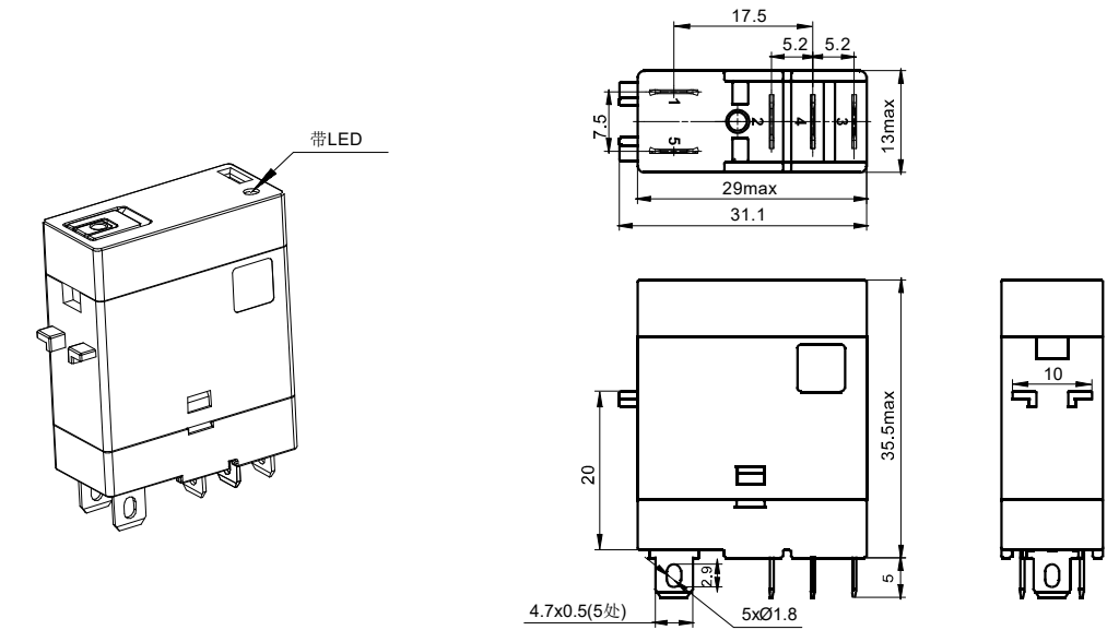
接线图 (底视图)
