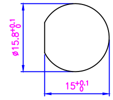
面板开孔尺寸
