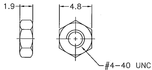
Nut: 2pcs
