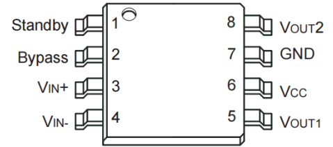
TS4871IST - MiniSO8
