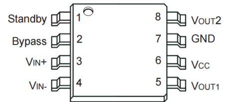
TS4871ID-TS4871IDT - SO8
