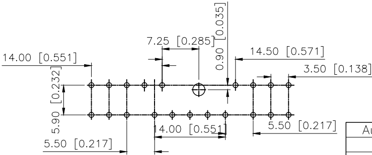
P.C.B LAYOUT
