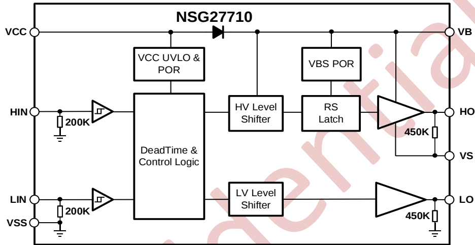
图 10-1 NSG27710 的功能框图
