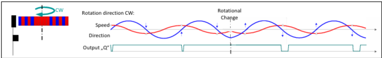
设置 “EDGE_POLAR = 1” 和 “FORWARD_DEF” = 0 的信号输出
