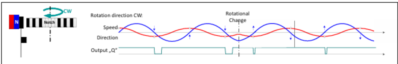
设置 “EDGE_POLAR = 0” 和 “FORWARD_DEF” = 0 时的信号输出
