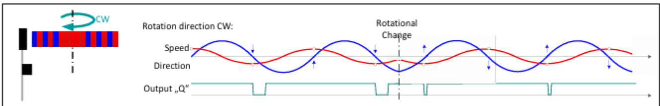
设置 “EDGE_POLAR = 1” 和 “FORWARD_DEF” = 1 的信号输出
