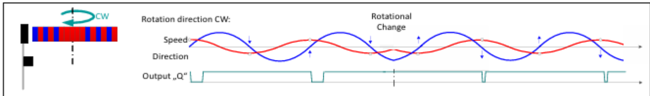
设置 “EDGE_POLAR = 0” 和 “FORWARD_DEF” = 1 的信号输出
