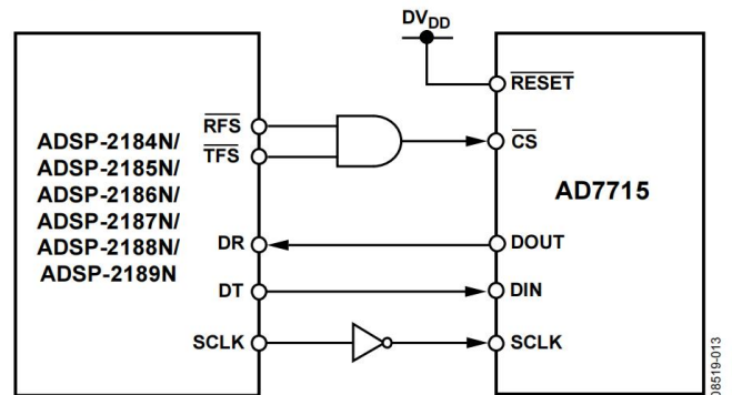
Figure 13. AD7715 to ADSP-2184N/ADSP-2185N/ADSP-2186N/ADSP-2187N/ADSP-2188N/ADSP-2189N Interface
