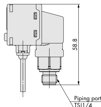
-B2L: TSJ1/4
