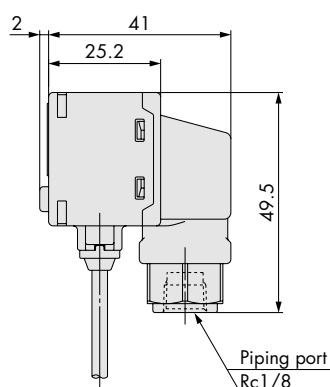
-C01L: Rc1/8
