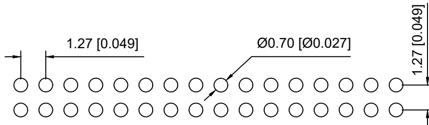
P.C.B LAYOUT
