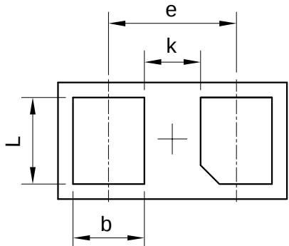
BOTTOM VVIEW
