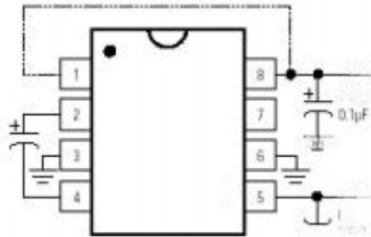
负电压转换(使用BOOST和LV)
