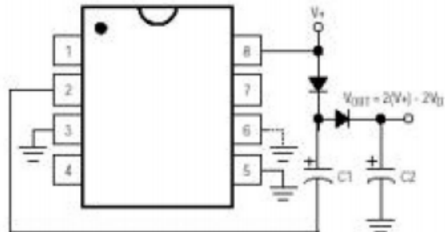
倍压输出电路
