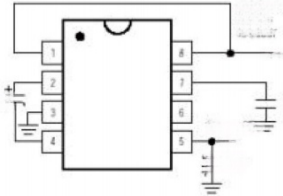
负电压转换(使用BOOST和 C_{osc} )
