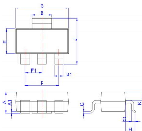
SOT-223-3L
