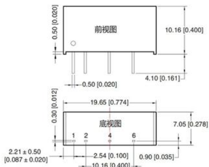
图4：外型尺寸
