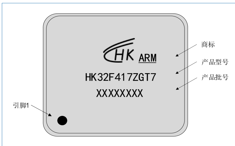
图 7-12 LQFP144 HK32F417ZGT7 丝印示例
