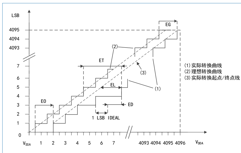
图 4-5 ADC 精度特征
