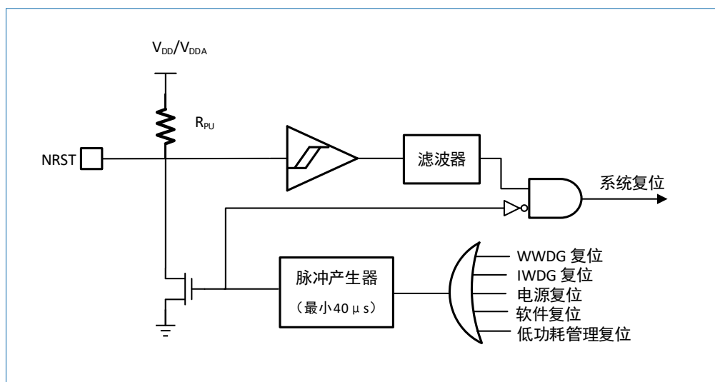
图 3-3 复位电路
