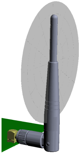
XZ-Plane Gain
