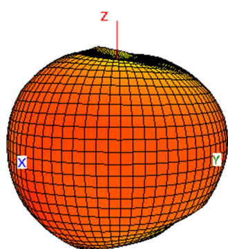
2400 MHz
