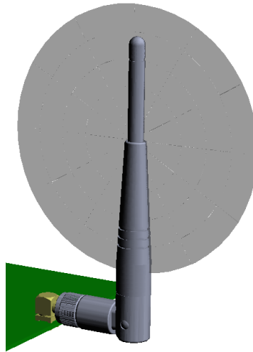
YZ-Plane Gain
