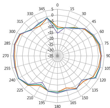
2450 MHz
